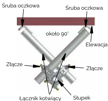
Przykład zakotwienia mogącego przenosić siły poziome
