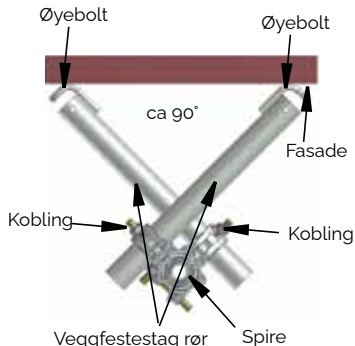
Eksempel på forankring som kan oppta horisontalkrefter
